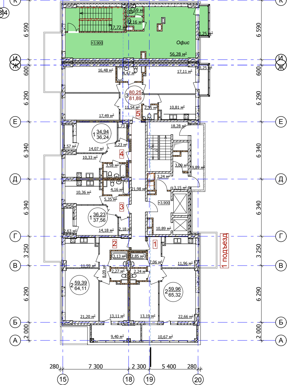
План 2 этажа на отм. +3.900
