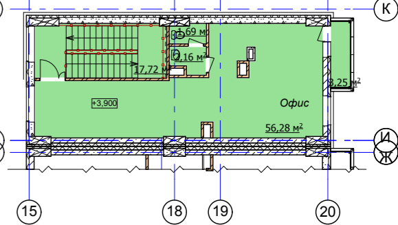
Фрагмент плана на отм. +3.900
