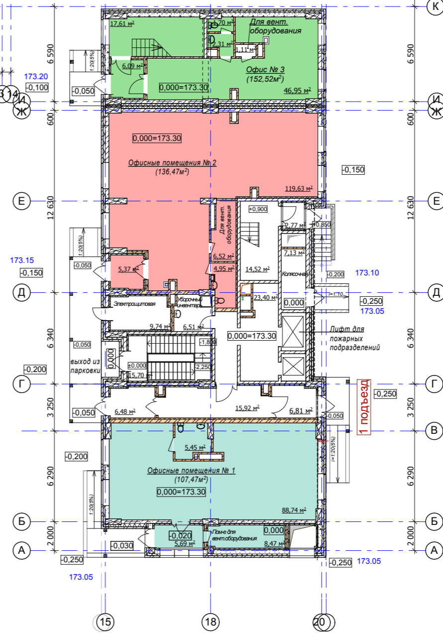
План 1 этажа на отм. 0.000
