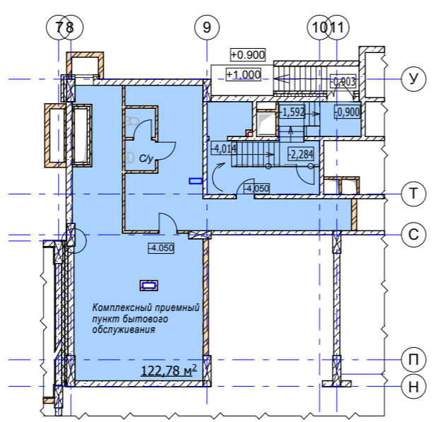
Фрагмент плана на отм. -4.050
